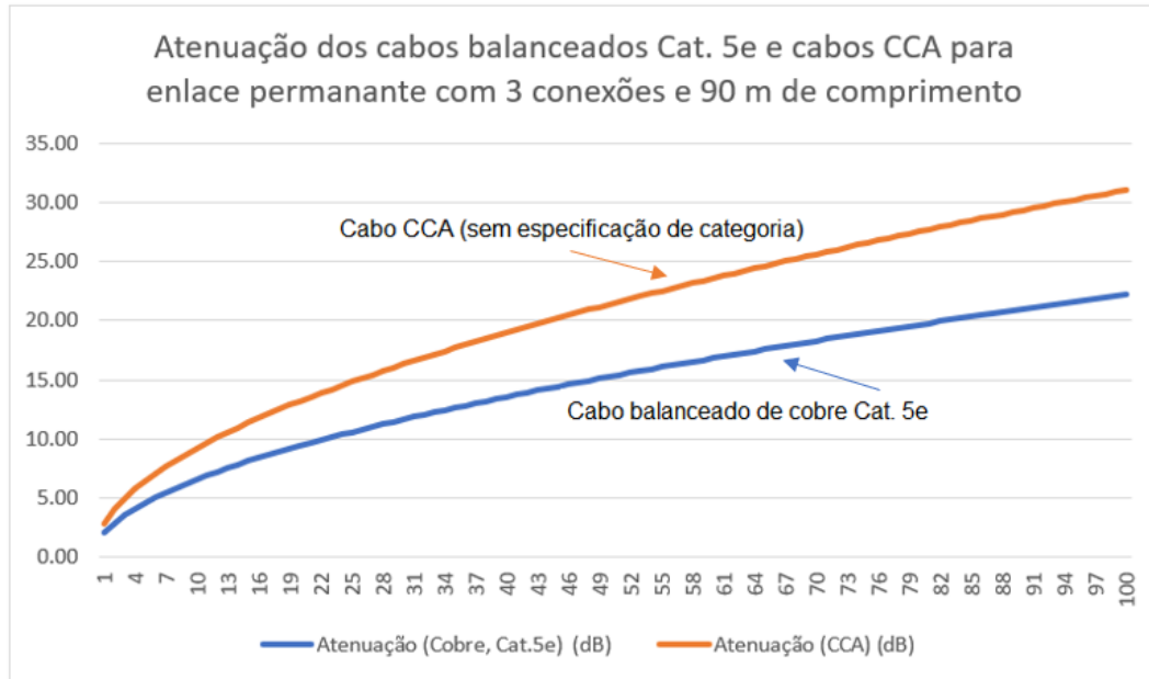
Figura 1 – Comparação entre as atenuações de cabos balanceados Cat. 5e e cabos CCA
