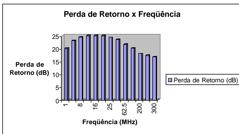
Figura 4 – Comportamento da perda de retorno em função da frequência para cabos de categorias 5e e 6
